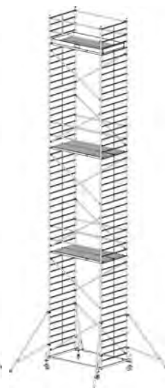
Arbeitshöhe: 14,40 m Gerüsthöhe: 13,40 m Standhöhe: 12,40 m
