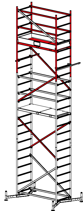
Grundgerüst Art.-No. 710116 + 1. Aufstockung Art.-No. 710130 + 2. Aufstockung Art.-No. 710154
