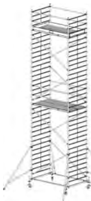
Arbeitshöhe: 10,40 m Gerüsthöhe: 9,40 m Standhöhe: 8,40 m
