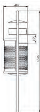
7031-52 Seitenansicht
