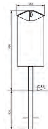
Frontansicht zum Einbetonieren
