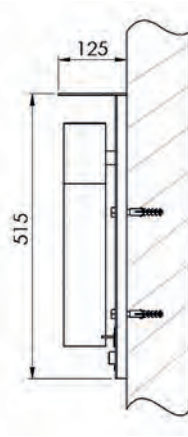
Modell 7061-01 Wandbefestigung
