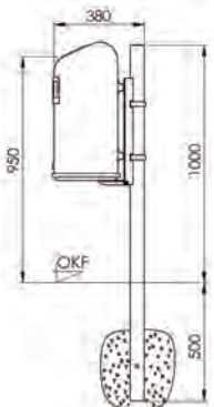
Pfostenbefestigung
