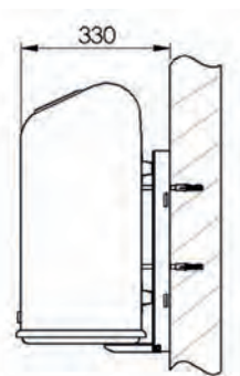
Wandbefestigung
