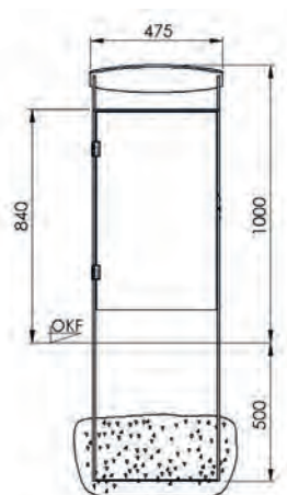
Frontansicht Ausführung zum Einbetonieren
