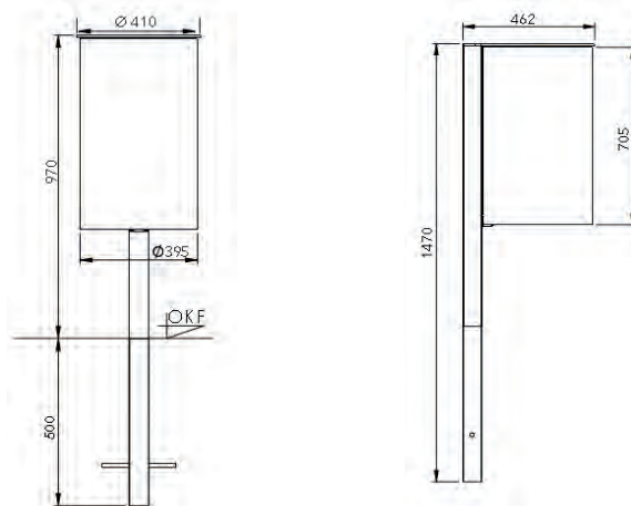
Frontansicht zum Einbetonieren
