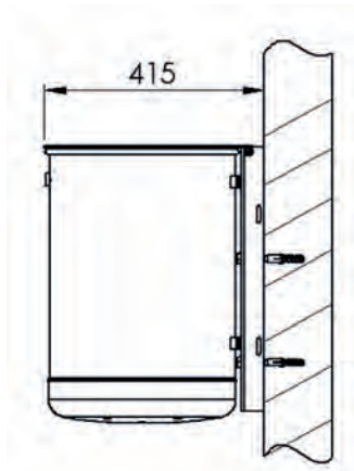
Wandbefestigung
