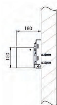
Wandbefestigung
