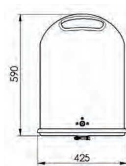
Frontansicht
