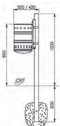
Pfostenbefestigung
