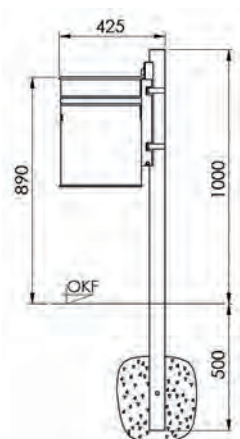
Pfostenbefestigung
