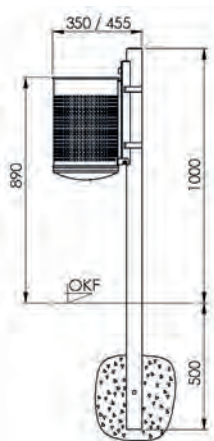
Pfostenbefestigung
