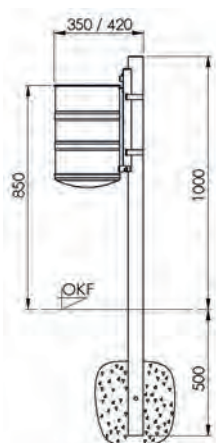
Pfostenbefestigung
