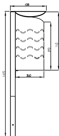
Seitenansicht zum Einbetonieren
