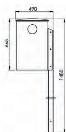
Seitenansicht
