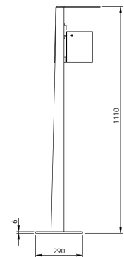
7070 S-00 Seitenansicht
