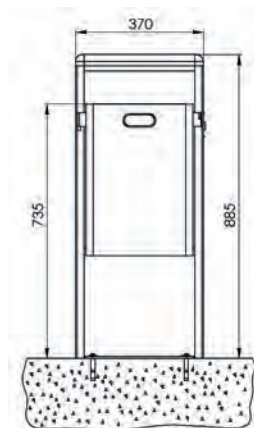
Frontansicht zum Aufschrauben 7083-30
