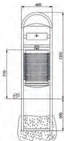
7031-52 Frontansicht Ausführung zum Einbetonieren
