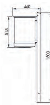
7039-15 Seitenansicht
