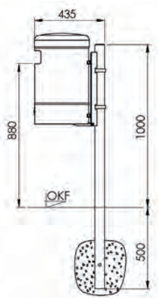
Pfostenbefestigung
