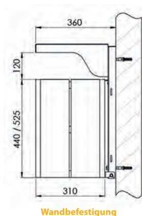
Wandbefestigung
