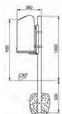
Pfostenbefestigung
