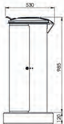
Seitenansicht 8059-00 zum Aufschrauben mit optionalem Betonsockel 7050-03
