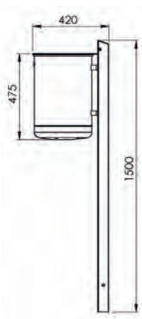
7038-15 Seitenansicht
