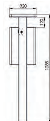
Seitenansicht zum Einbetonieren 7083-70
