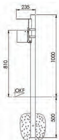
Pfostenbefestigung
