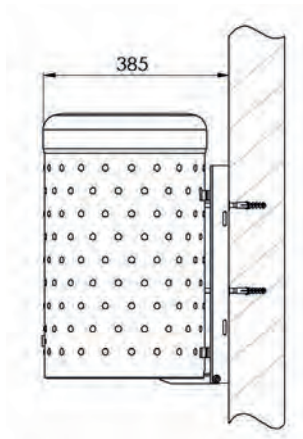
Wandbefestigung
