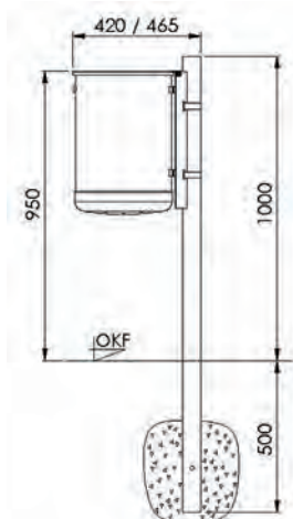
Pfostenbefestigung
