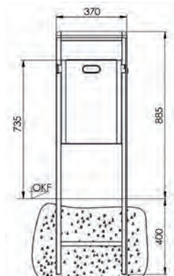
Frontansicht zum Einbetonieren 7083-70
