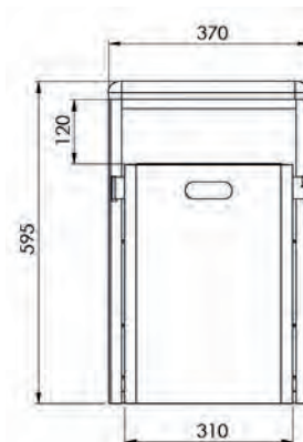
Frontansicht
