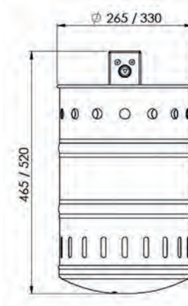
Frontansicht
