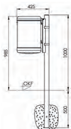
Pfostenbefestigung
