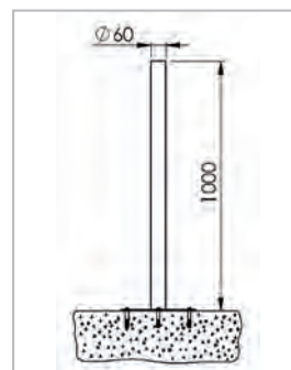
Abb.: Montageempfehlung Pfosten zum Aufschrauben
