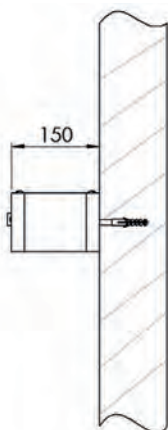
Modell 7068-00 Wandbefestigung
