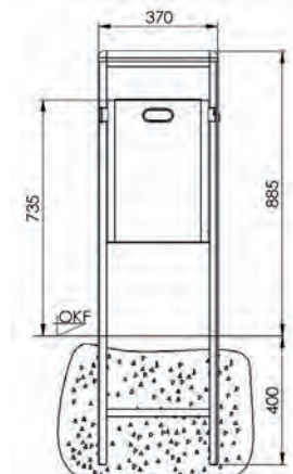
Frontansicht zum Einbetonieren 7083-40
