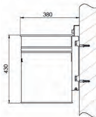
Wandbefestigung
