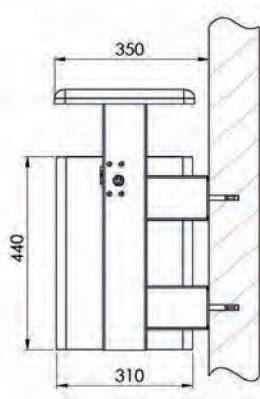
Wandbefestigung
