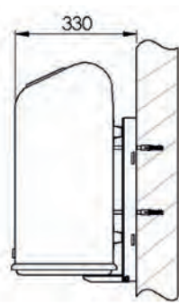
Wandbefestigung
