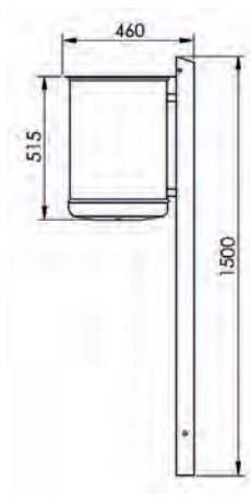
Seitenansicht
