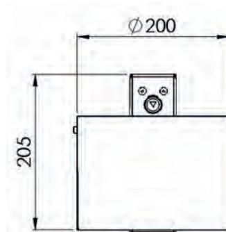
Frontansicht
