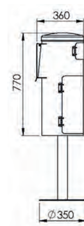
7077-01 Seitenansicht
