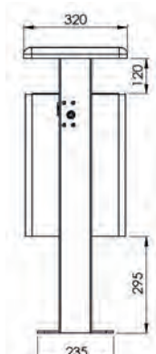
Seitenansicht zum Aufschrauben 7083-60
