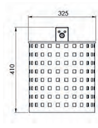
Frontansicht
