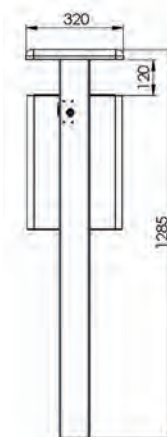
Seitenansicht zum Einbetonieren 7083-40
