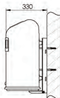
Wandbefestigung
