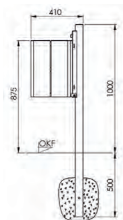
Pfostenbefestigung
