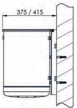
Wandbefestigung
