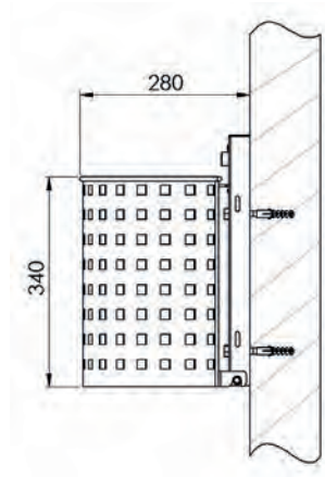
Wandbefestigung
