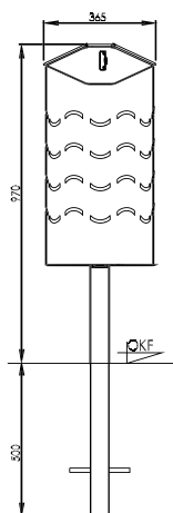
Frontansicht zum Einbetonieren
