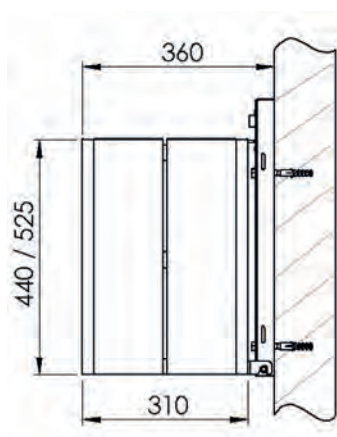
Wandbefestigung
