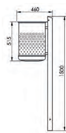
7039-00 Seitenansicht
