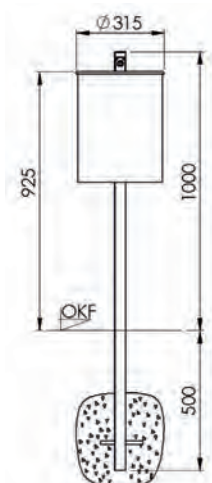
Frontansicht
