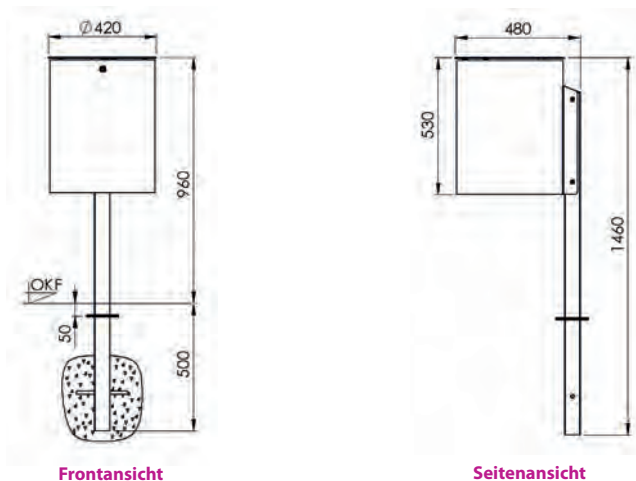
Frontansicht
