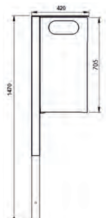
Seitenansicht zum Einbetonieren
