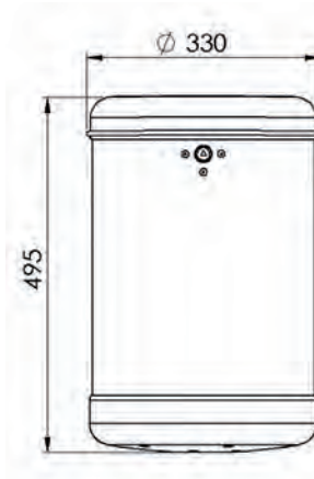
Frontansicht
