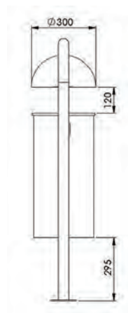
Seitenansicht
