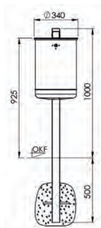
7038-15 Frontansicht
