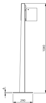
7067 S-00 Seitenansicht
