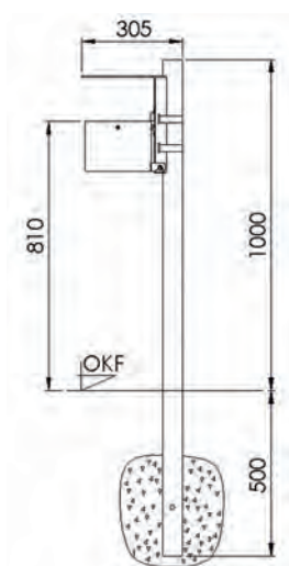
Pfostenbefestigung
