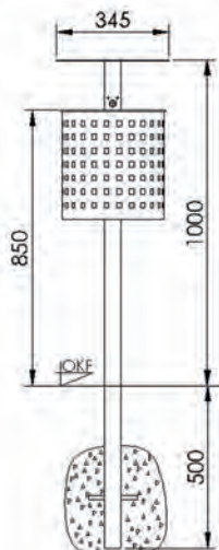
Frontansicht Ausführung zum Einbetonieren
