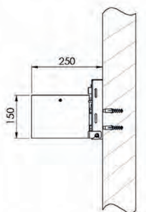
Wandbefestigung
