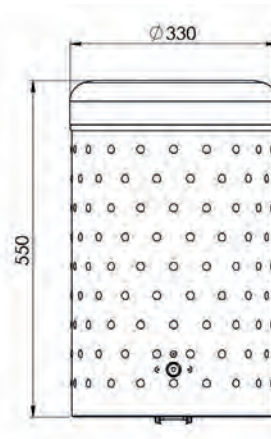
Frontansicht
