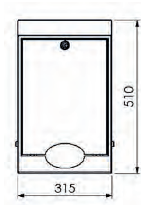
Frontansicht
