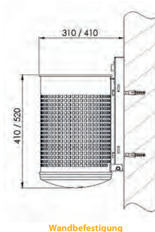
Wandbefestigung
