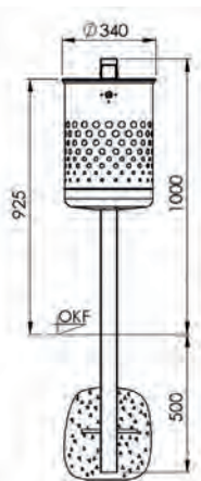
7038-00 Frontansicht
