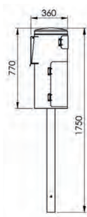
7077-00 Seitenansicht
