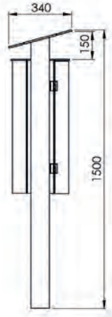
Seitenansicht
