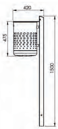
7038-00 Seitenansicht
