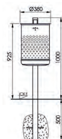
7039-00 Frontansicht
