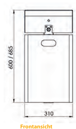
Frontansicht
