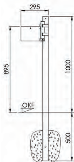
Pfostenbefestigung
