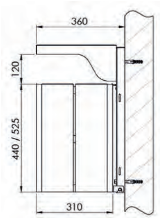
Wandbefestigung
