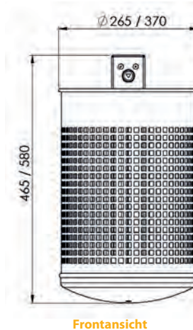
Frontansicht
