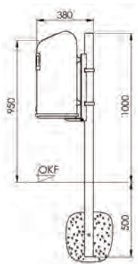
Pfostenbefestigung
