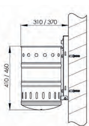
Wandbefestigung
