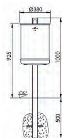
7039-15 Frontansicht
