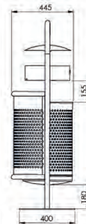
7031-62 Seitenansicht
