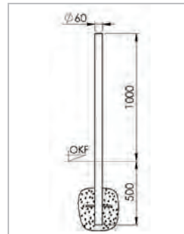
Abb.: Montageempfehlung Pfosten zum Einbetonieren
