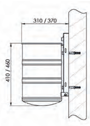
Wandbefestigung
