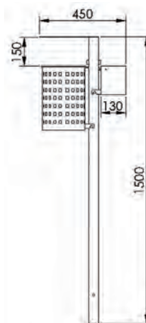
Seitenansicht
