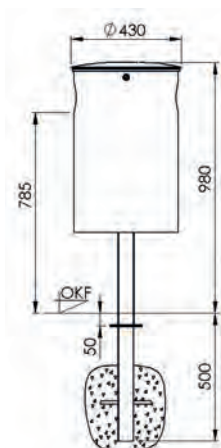
Frontansicht
