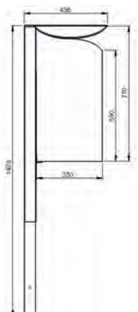
Seitenansicht zum Einbetonieren
