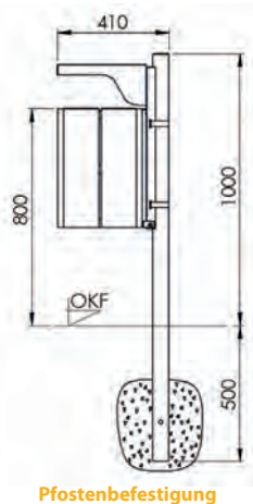
Pfostenbefestigung
