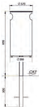
Frontansicht zum Einbetonieren
