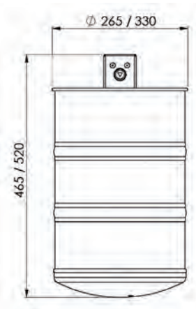
Frontansicht
