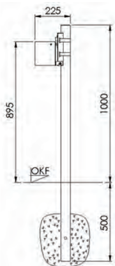
Pfostenbefestigung
