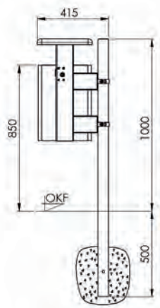
Pfostenbefestigung
