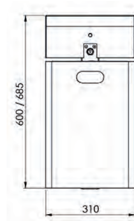
Frontansicht
