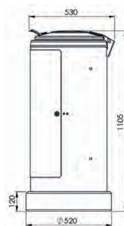
Montage auf optionalem Betonsockel 7050-03
