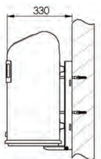
Wandbefestigung
