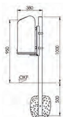
Pfostenbefestigung
