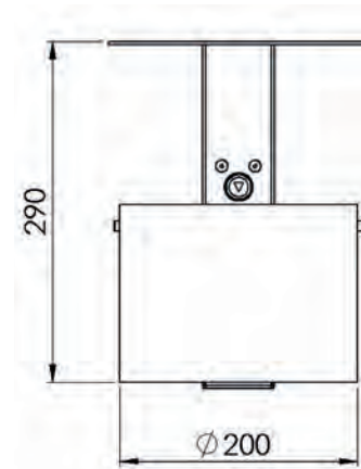
Frontansicht
