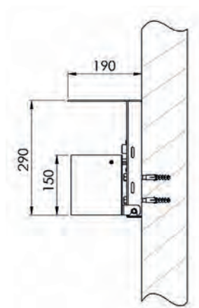
Wandbefestigung
