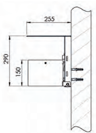
Wandbefestigung
