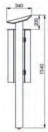
Seitenansicht
