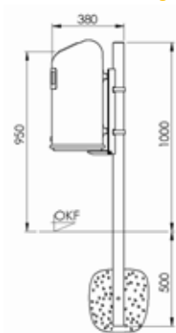
Pfostenbefestigung
