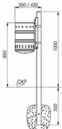
Pfostenbefestigung
