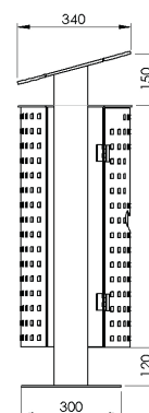
Seitenansicht
