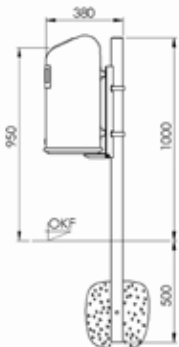
Pfostenbefestigung
