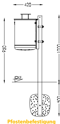
Pfostenbefestigung
