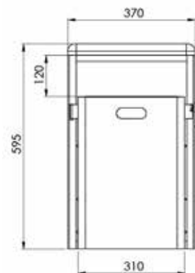
Frontansicht
