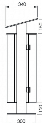
Seitenansicht
