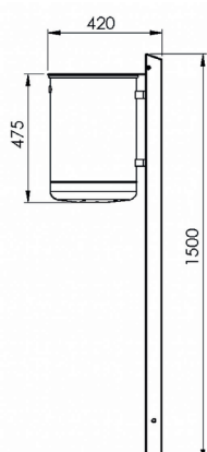
7038-15 Seitenansicht
