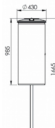
Vorderansicht 8059-01 zum Einbetonieren
