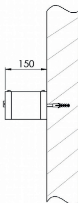
Modell 7068-00 Wandbefestigung
