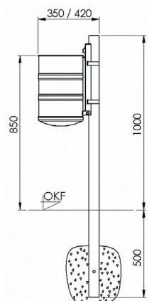
Pfostenbefestigung
