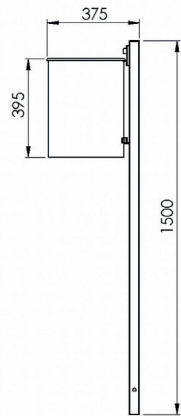
Seitenansicht
