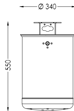
Frontansicht
