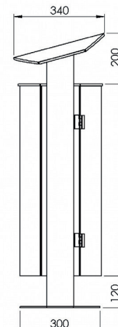
Seitenansicht
