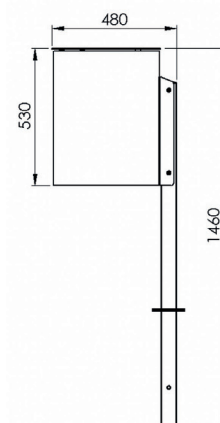
Seitenansicht
