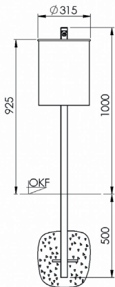
Frontansicht
