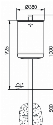
7039-15 Frontansicht
