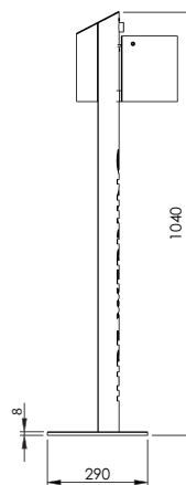
7067 S-01 Seitenansicht
