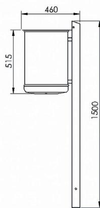
Seitenansicht
