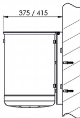
Wandbefestigung
