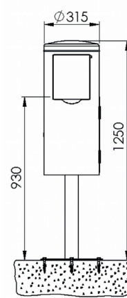
7077-01 Frontansicht zum Aufschrauben
