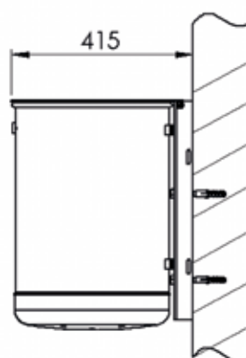
Wandbefestigung
