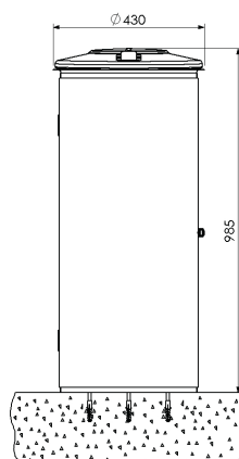
Vorderansicht 8059-10 zum Aufschrauben
