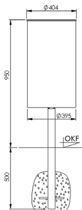
Frontansicht zum Einbetonieren
