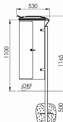
Seitenansicht 8059-01 zum Einbetonieren
