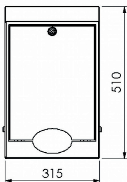
Frontansicht
