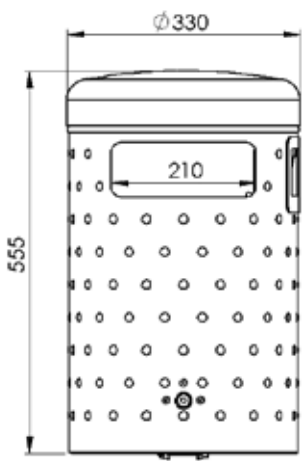
Frontansicht
