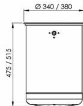
Frontansicht
