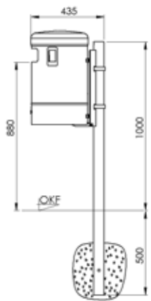
Pfostenbefestigung
