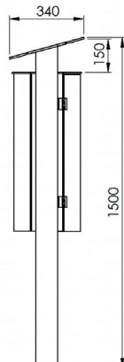
Seitenansicht
