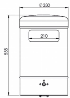
Frontansicht
