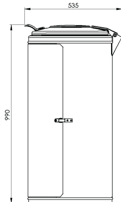
Seitenansicht
