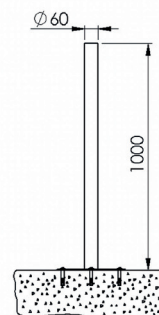
Abb.: Montageempfehlung Pfosten zum Aufschrauben
