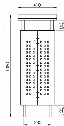
Seitenansicht
