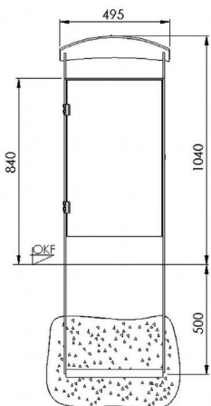
Frontansicht Ausführung zum Einbetonieren
