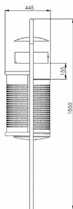
7031-52 Seitenansicht
