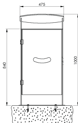
Frontansicht Ausführung zum Aufschauben
