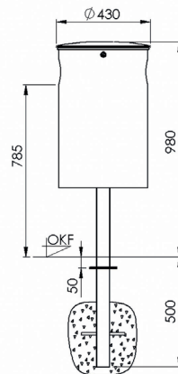
Frontansicht
