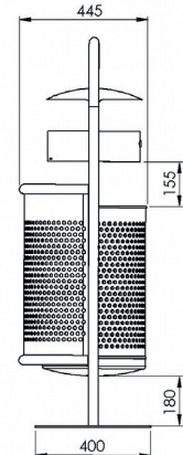
7031-62 Seitenansicht
