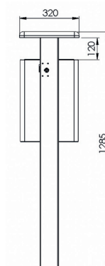
Seitenansicht zum Einbetonieren 7083-70
