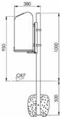
Pfostenbefestigung
