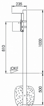
Pfostenbefestigung
