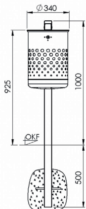
7038-00 Frontansicht
