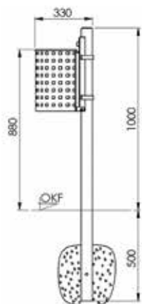
Pfostenbefestigung
