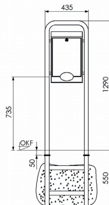
Frontansicht
