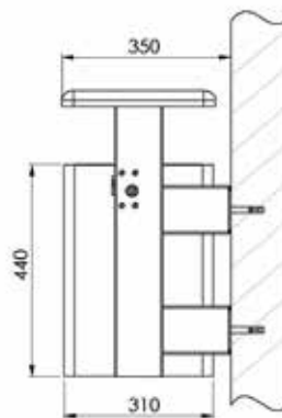
Wandbefestigung
