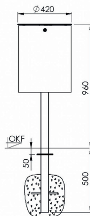
Frontansicht
