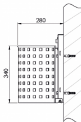
Wandbefestigung
