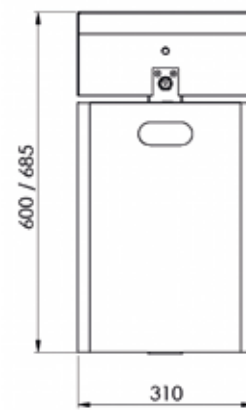
Frontansicht
