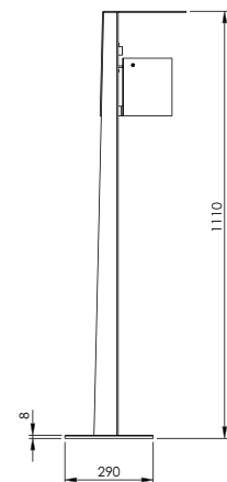
7070 S-00 Seitenansicht
