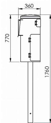
7077-00 Seitenansicht
