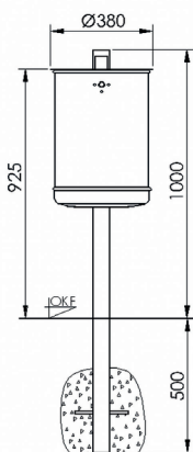
Frontansicht
