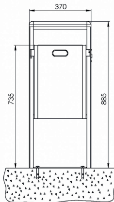
Frontansicht zum Aufschrauben 7083-30
