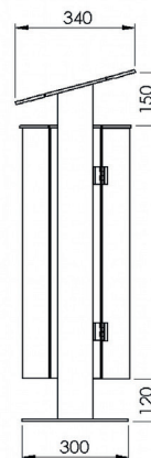
Seitenansicht
