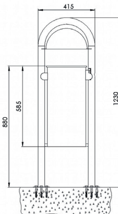
Frontansicht Ausführung zum Aufschrauben
