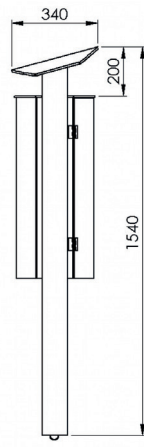
Seitenansicht
