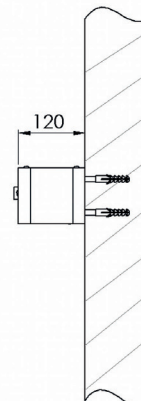
Modell 7068-10 Wandbefestigung
