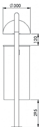
Seitenansicht
