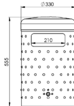
Frontansicht
