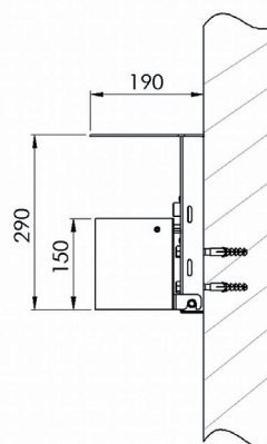
Wandbefestigung
