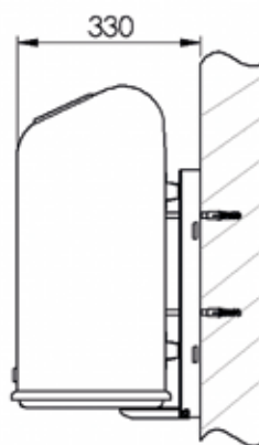
Wandbefestigung
