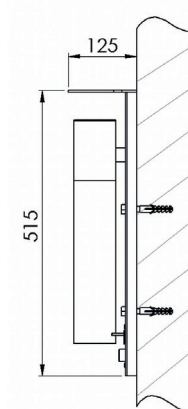
Modell 7061-01 Wandbefestigung
