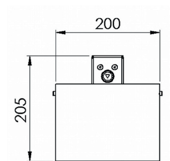
Frontansicht
