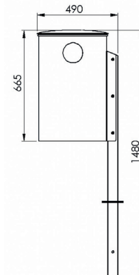
Seitenansicht
