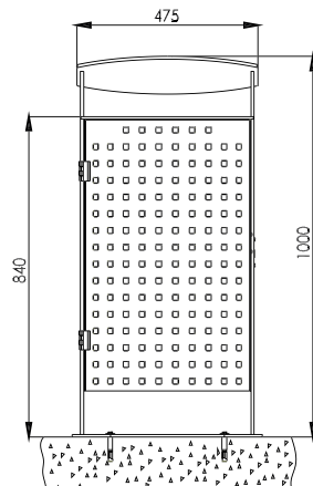
Frontansicht Ausführung zum Aufschauben
