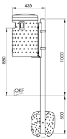
Pfostenbefestigung
