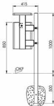
Pfostenbefestigung
