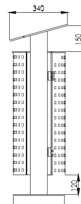
Seitenansicht
