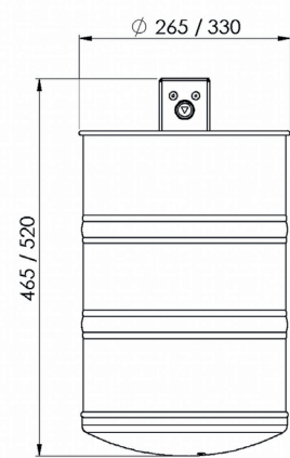
Frontansicht
