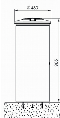
Vorderansicht 8059-00 zum Aufschrauben
