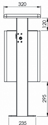
Seitenansicht zum Aufschrauben 7083-30
