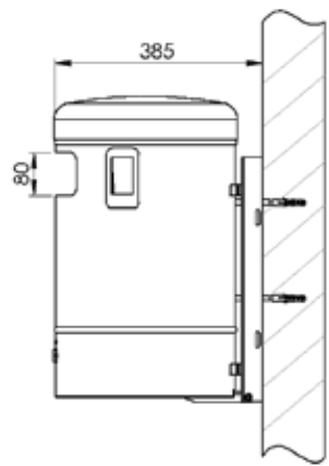
Wandbefestigung
