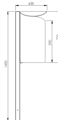
Seitenansicht zum Einbetonieren
