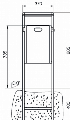
Frontansicht zum Einbetonieren 7083-40
