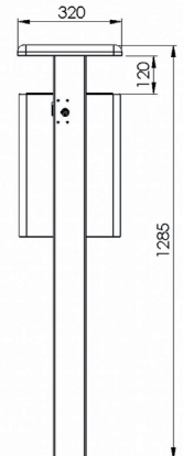
Seitenansicht zum Einbetonieren 7083-40
