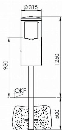
7077-00 Frontansicht zum Einbetonieren
