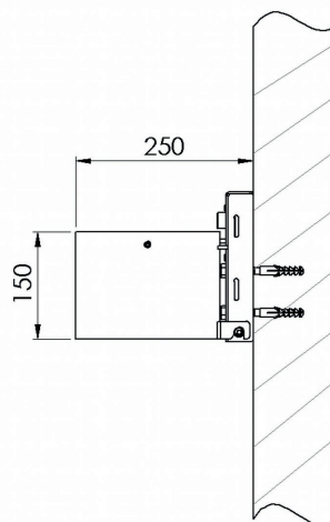
Wandbefestigung
