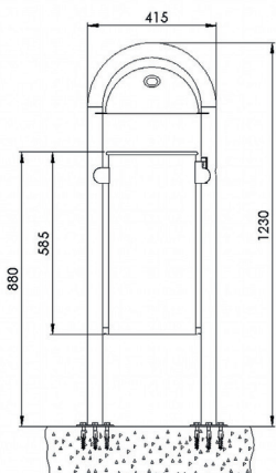
Frontansicht Ausführung zum Aufschauben
