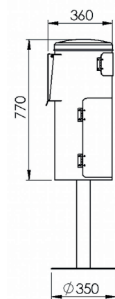
7077-01 Seitenansicht
