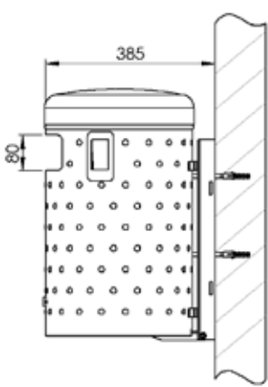
Wandbefestigung
