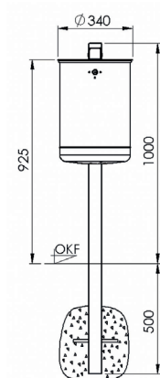
7038-15 Frontansicht
