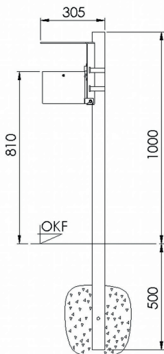
Pfostenbefestigung
