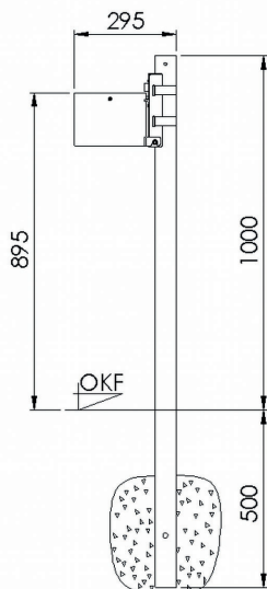
Pfostenbefestigung
