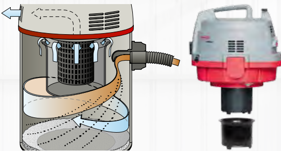
Die Grafik zeigt das patentierte Wasser-Abscheidesystem
